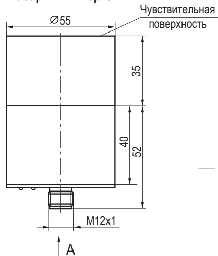
Габаритный чертёж
